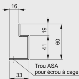
Profil de montage 19"
