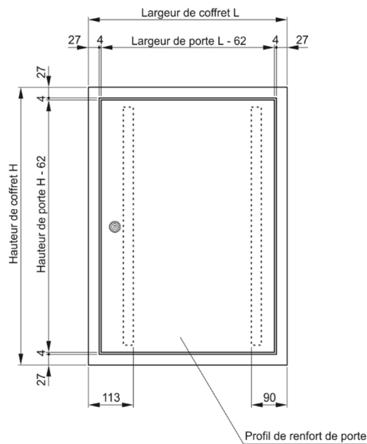
Hauteur de 400 à 849 mm, porte simple
