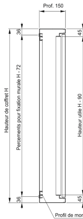
Coupe B-B (prof. 150 mm)
