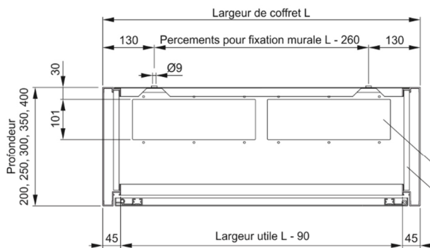
Coupe A-A: avec fente d'introduction (prof. 200-400 mm)
