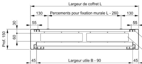
Coupe A-A: avec fente d'introduction (prof. 150 mm)
