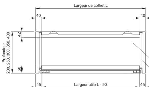
Coupe A-A: ouvert en bas (prof. 200-400 mm)
