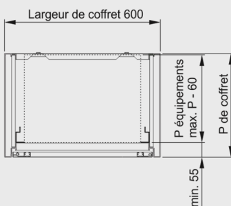
Coupe A-A
