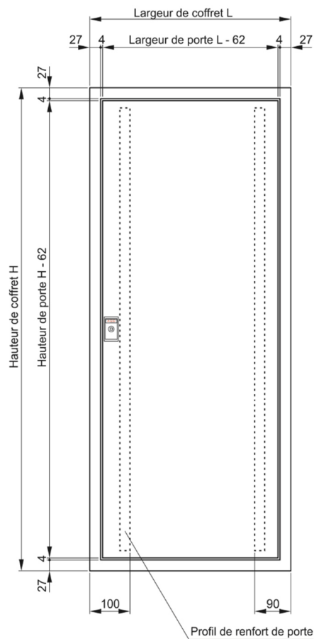
Hauteur de 850 à 2200 mm, porte simple
