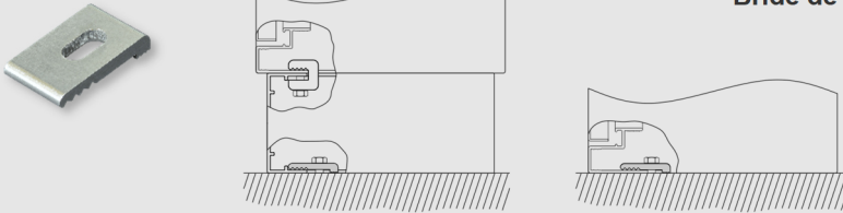
Bride de fixation au sol
