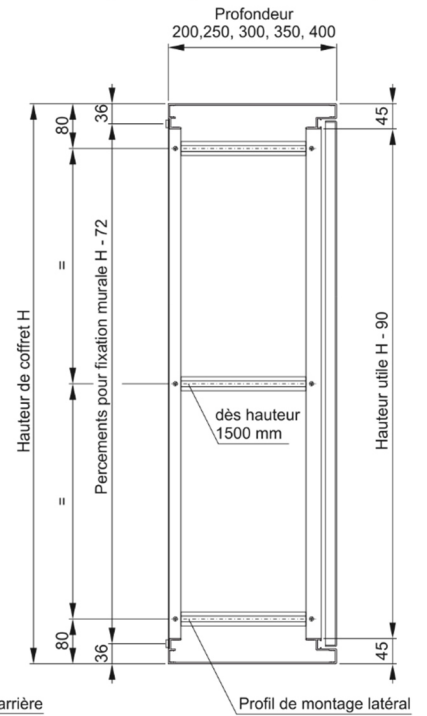
Coupe B-B (prof. 200-400 mm)
