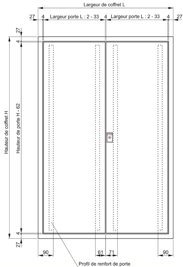
Hauteur de 400 à 2200 mm, porte double
